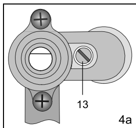
13 Regulační šroub pro minimální tepelný výkon
